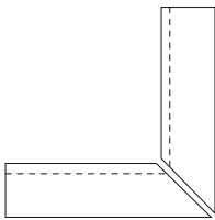
ÁNGULO PELDAÑO RECTO 120. INT. ANTISLIP 120 x 33 x 45/3 (G 46 x 2) 48" x 13" x 17,7"/1" ♦
