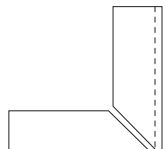
ÁNGULO PELDAÑO RECTO EXT. 61,3 x 32 x 46/3 (G 56 x 2) 24" x 12,5" x 18"/1"
