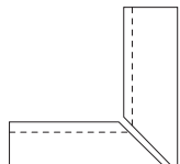
ÁNGULO PELDAÑO RECTO INT. 61,3 x 32 x 46/3 (G 56 x 2) 24" x 12,5" x 18"/1"
