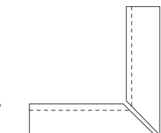
ÁNGULO PELDAÑO 120. INT ANTISLIP 120 x 32 x 45/3 (G 46 x 2) 48" x 12,5" x 17,7"/1"
