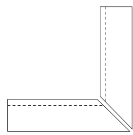
ÁNGULO PELDAÑO 120 INT. ANTISLIP 120 x 33 x 45/3 (G 46 x 2) 48" x 13" x 17,7"/1" ♦
